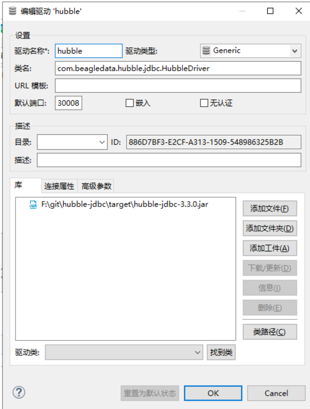
图 2: jdbc
